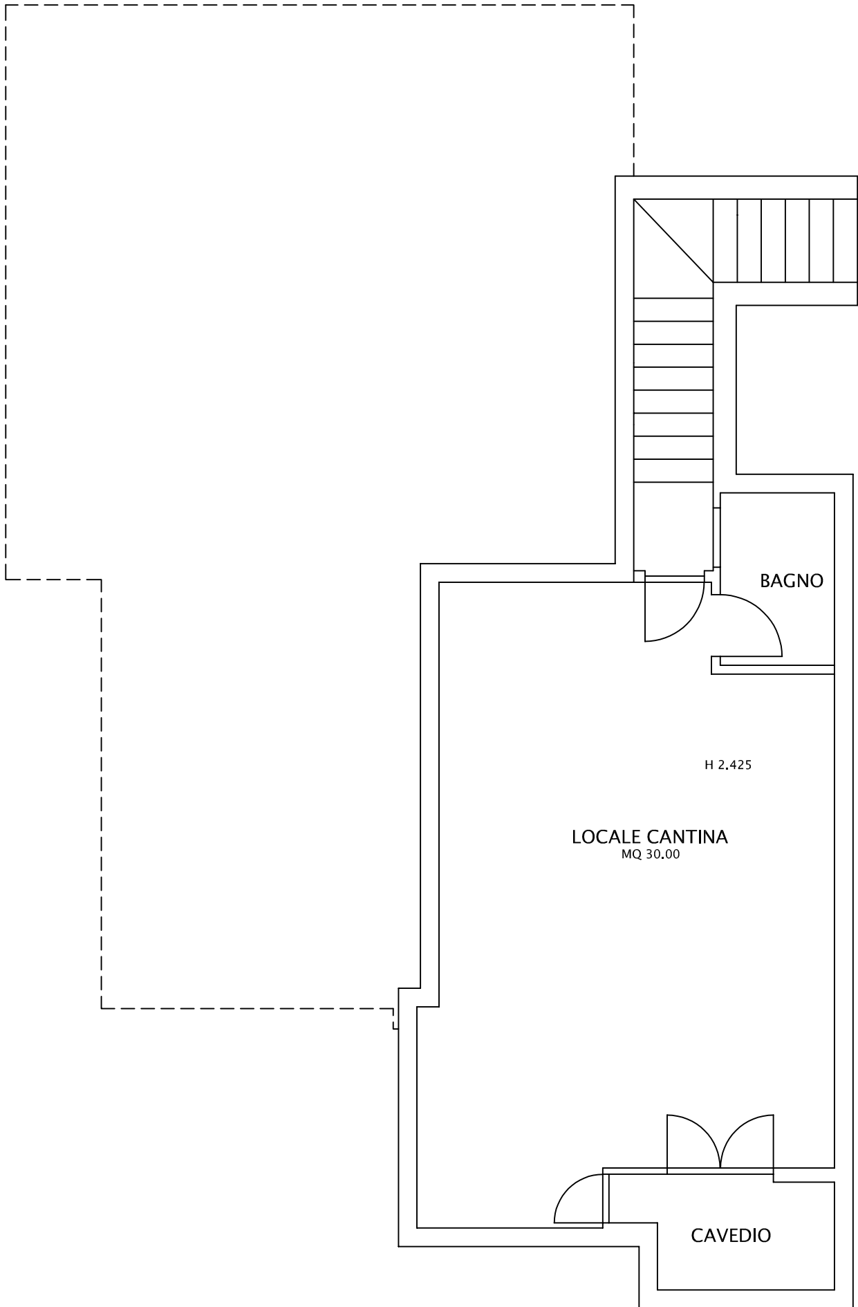
PIANTA PIANO INTERRATO CASA "A"
