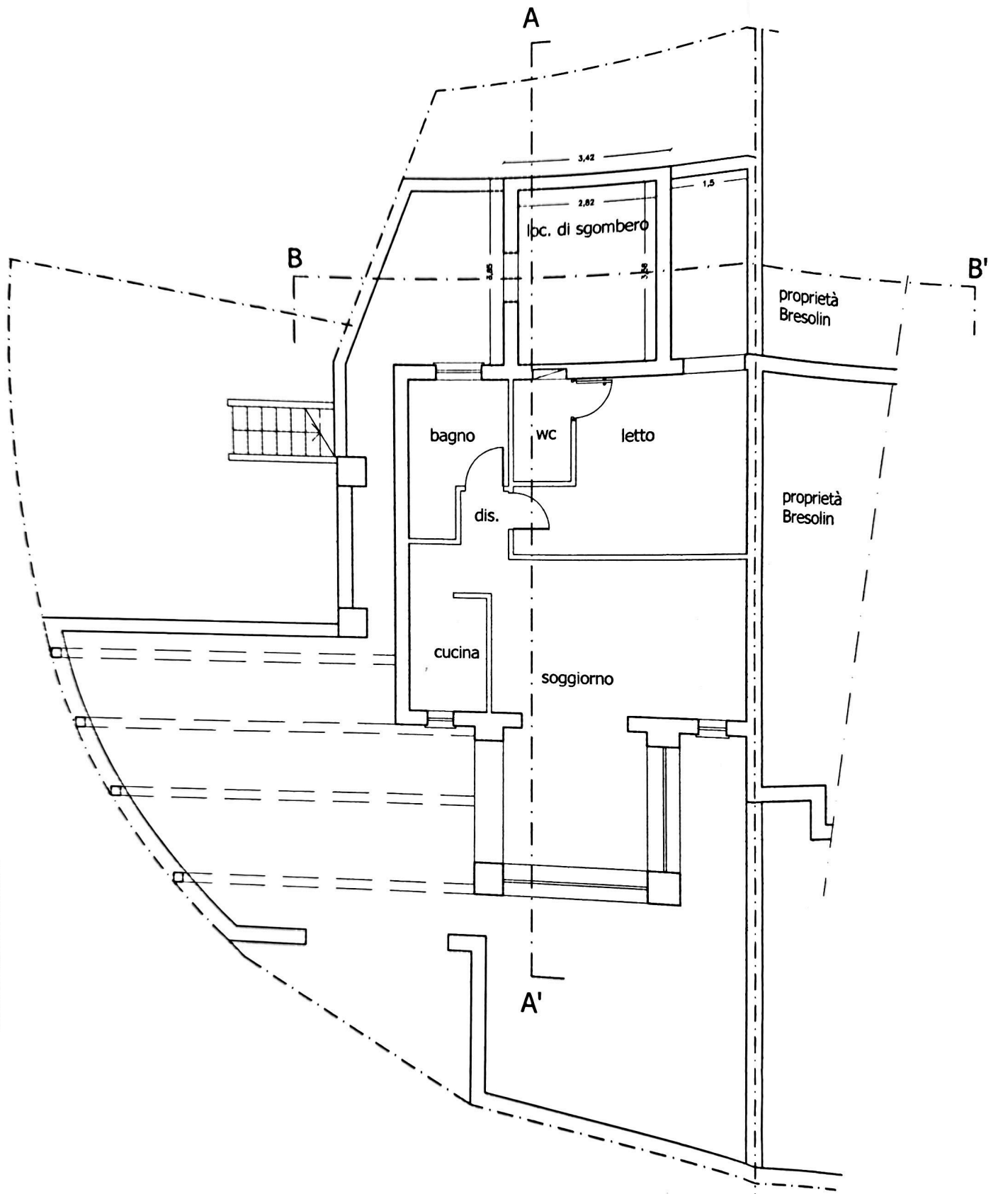
PIANTA DEL PIANO TERRA STATO ATTUALE
