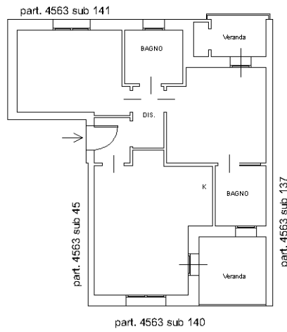
PIANO TERRA H. 2,70
