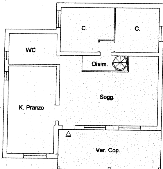
PIANTA PIANO TERRA H. MT. 2.80
