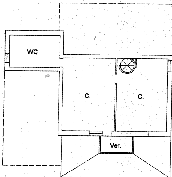
PIANTA PIANO PRIMO H. MT. 2.40
